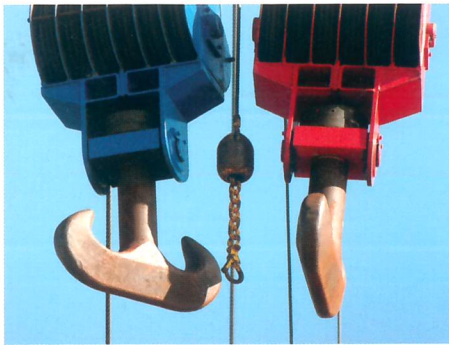
大容量 油壓 Hook Block (20 ton~500 ton)
